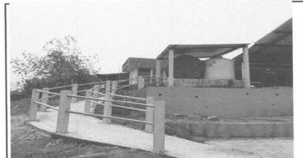
Foto 4: RAMPA BARANDEADA
